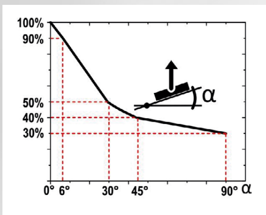
Løftekapasitetsendringer ved vinkling av lasten. TML 90 R
